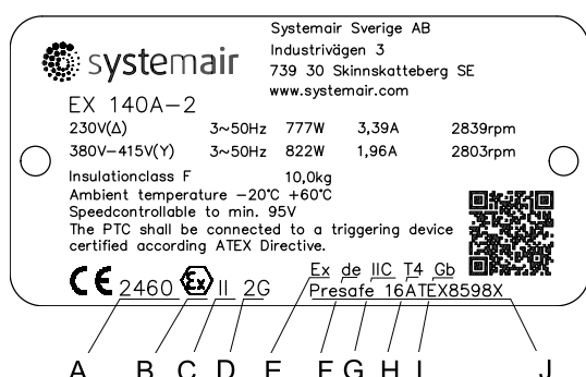
Рис. 4 Заводская табличка
